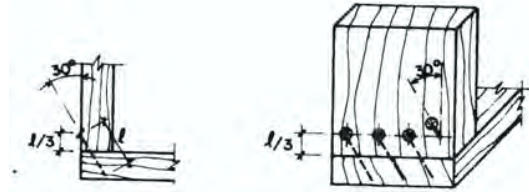
Fig. 10.2.4.1c. Ubicación de clavos lanceros.
