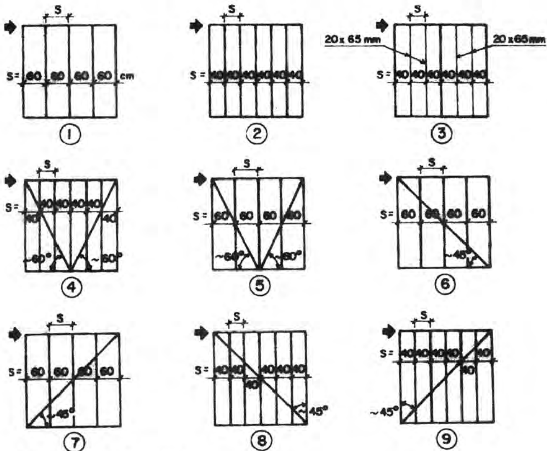
Fig. 8.6.1. Tipos de entramados
