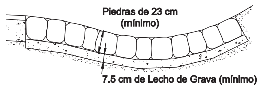
CUNETA DE CANTOS RODADOS
