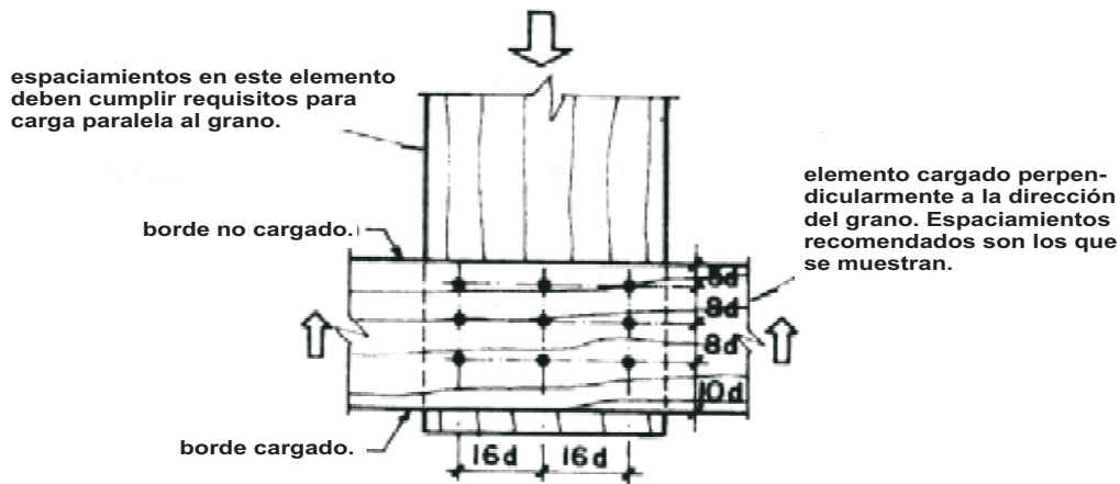
Fig. 10.2.5.2b. Elemento cargados perpendicularmente al grano
