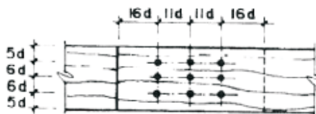
Fig. 10.2.5.3a. Elemento cargados paralelamente al grano
