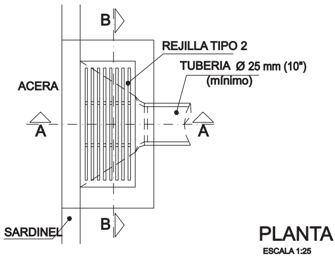
FIGURA N° 7 SUMIDERO CHICO CONECTADO A LA CAMARA - S3
