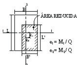
(B) ÁREA REDUCIDA - CIMIENTO RECTANGULAR
