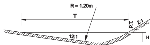
CUNETA ASFÁLTICA
