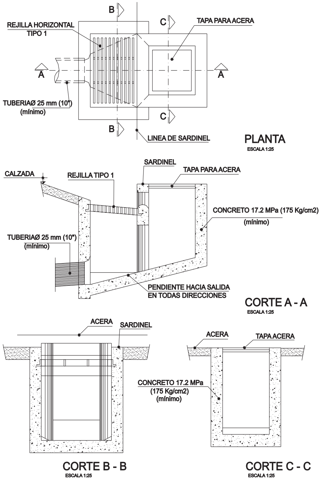
FIGURA N° 6 SUMIDERO TIPO GRANDE CONECTADO A TUBERIA – S2
