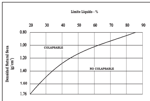
FIGURA 7 CRITERIOS DEL POTENCIAL DE COLAPSO
