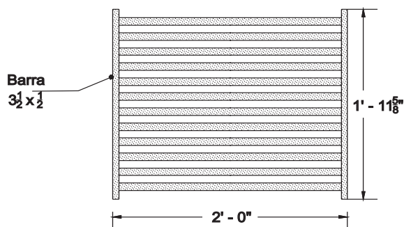
Fig. N° 12 REJILLA CUADRADA
