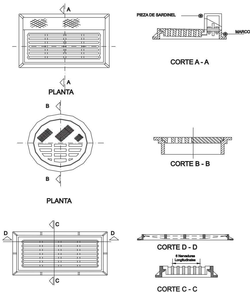
FIGURA N° 9 REJILLAS DE FIERRO FUNDIDO PARA SUMIDEROS
