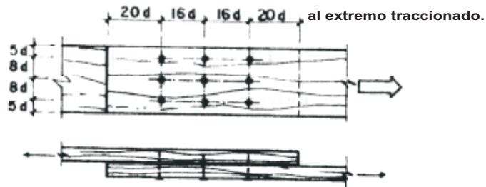
Fig. 10.2.5.2a. Elemento cargados paralelamente al grano
