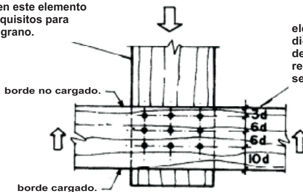
Fig. 10.2.5.3b. Elemento cargados perpendicularmente al grano
