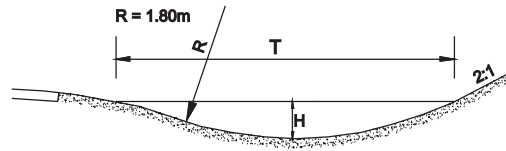
CUNETA SEGMENTAL
