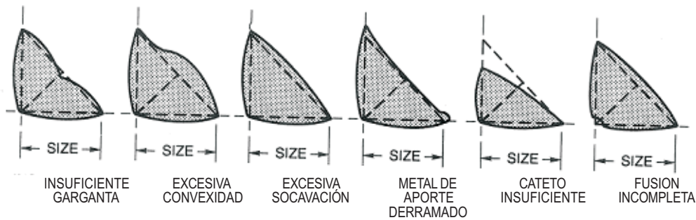
C) Perfiles de Soldadura de Filete Inaceptables
