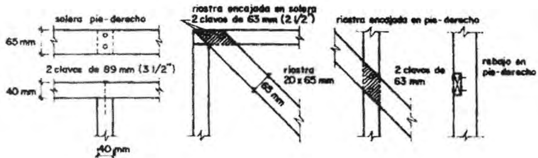
TODOS LOS PIE - DERECHOS Y SOLERAS DE 40 x 65mm EXCEPTO DONDE SE INDICA, RIOSTRAS DE 20 X 65 mm
