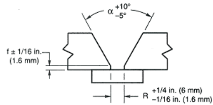
B) SOLDADURA POR CANAL CON RESPALDO - FONDO NO RANURADO POR LA PARTE POSTERIOR
