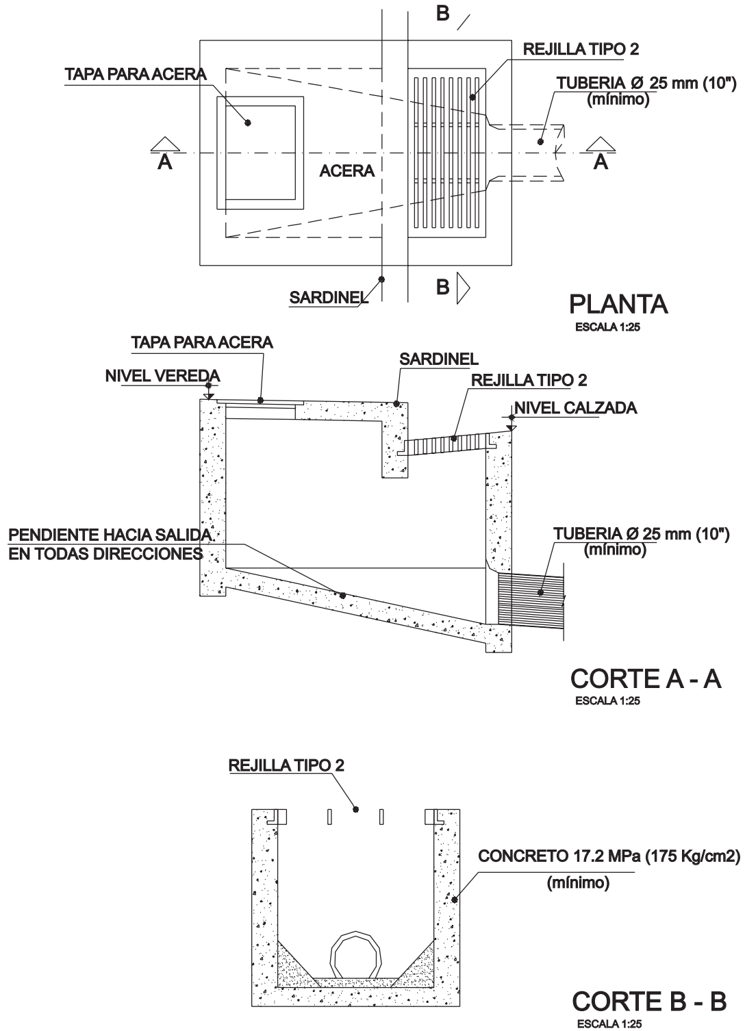
FIGURA N° 8 SUMIDERO TIPO CHICO CONECTADO A LA TUBERÍA- S4
