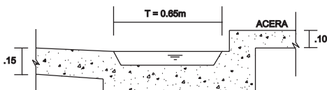
CUNETA TRAPEZOIDAL
