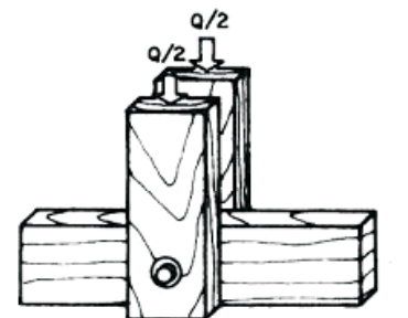
Carga Q (b) cargas perpendiculares al grano en los elementos central y paralelos al grano en los elementos laterales.
