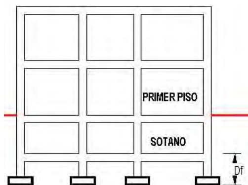
PROFUNDIDAD DE CIMENTACIÓN (D f ) EN ZAPATAS BAJO SÓTANO
