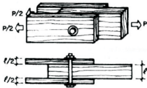
Fig. 10.3.2.2a Unión emperrada a doble cizallamiento cargas paralelas al grano en todos los elementos (Carga P).
