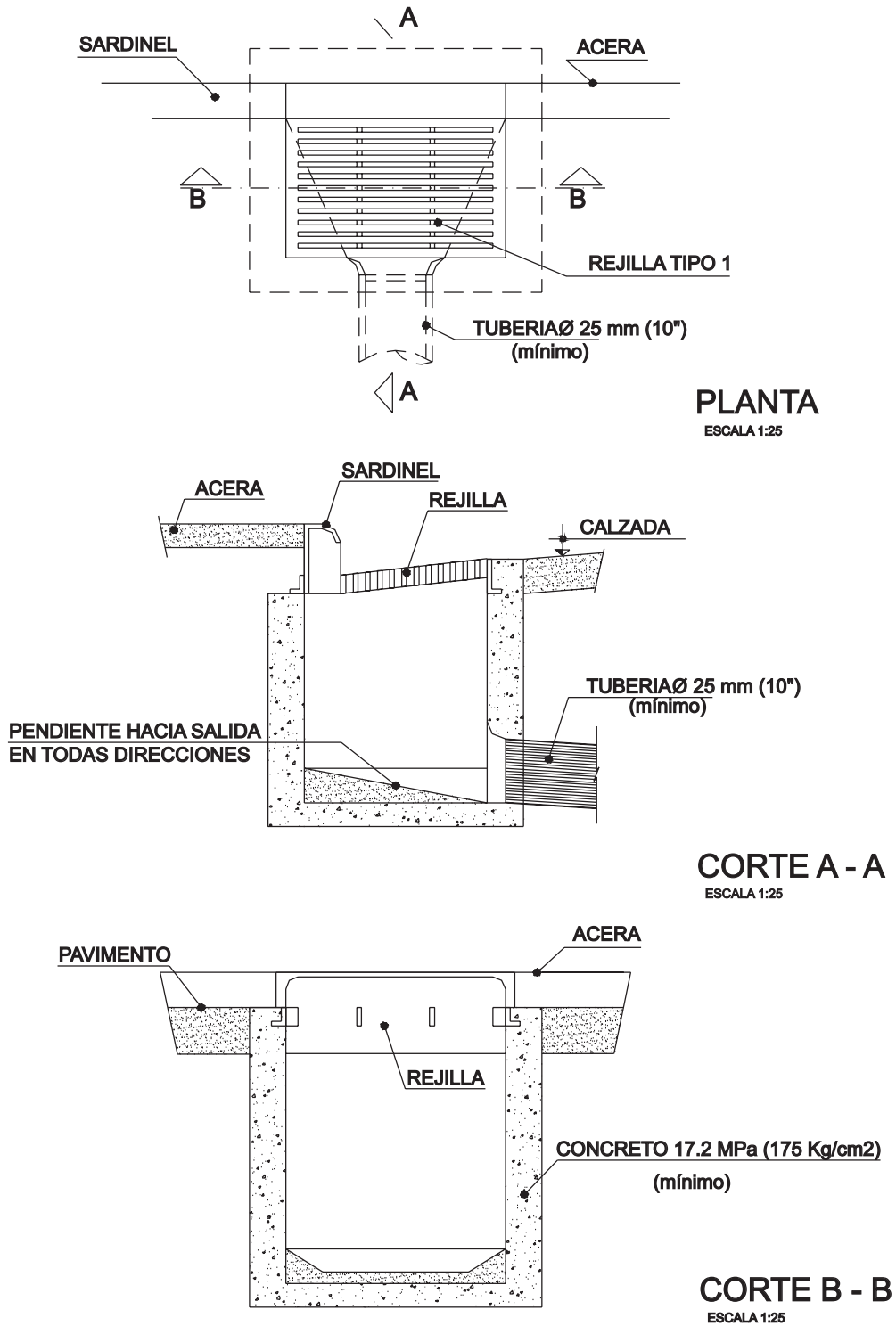
FIGURA N° 5 SUMIDERO GRANDE CONECTADO A CÁMARA – S1
