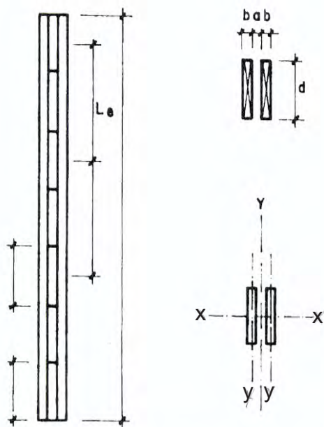
Fig. 7.9.1. Columna compuesta por dos piezas separadas por bloques.
