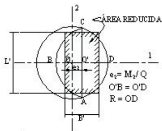
(C) ÁREA REDUCIDA - CIMIENTO CIRCULAR
