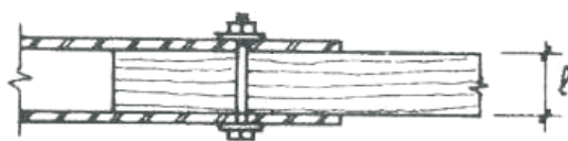
Fig. 10.3.2.4. Unión emperrada con pletinas metálicas
