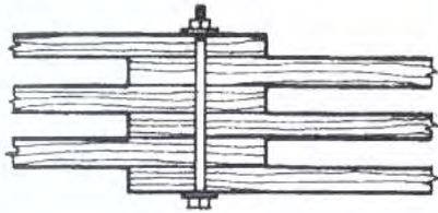
Fig. 10.3.2.6. Unión empernada sometida a cizallamiento múltiple
