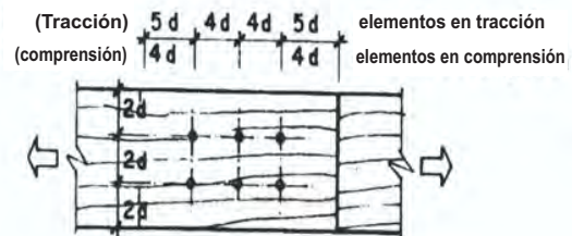
Fig. 10.3.3.3a Espaciamientos mínimos entre pernos, cargas paralelas al grano.
