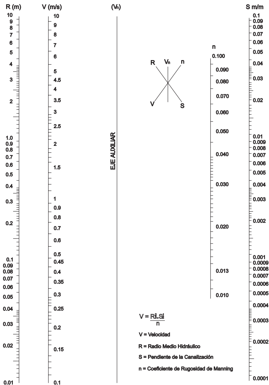
GRÁFICO N° 1 NOMOGRAMA PARA LA SOLUCIÓN DE LA ECUACIÓN DE MANNING
