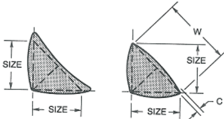
A) Perfiles de Soldadura de Filete Deseables
