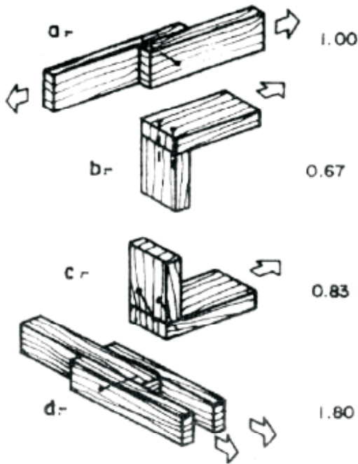
Fig. 10.2.3.1. Factores modificatorios de las cargas admisibles para uniones clavadas sometida a cizallamiento simple
