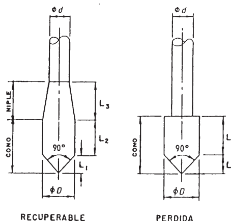
FIG. 9 Alternativas de cono
