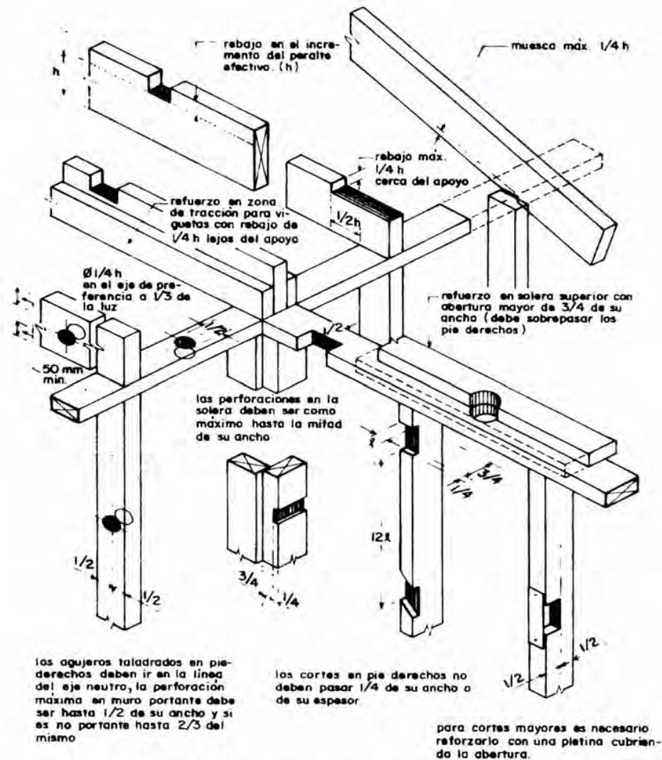
Fig. 12.2.2 Perforaciones y rebajos en elementos de madera.
