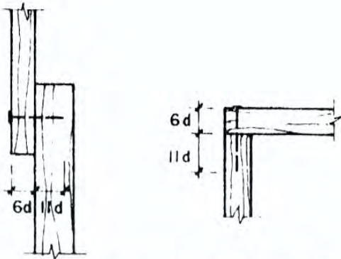
Fig. 10.2.4.1a. Espesores mínimos y penetración de clavos sometidos a cizallamiento simple
